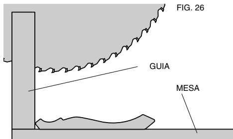
LA MOLDURA PLANA EN LA MESA Y CONTRA LA GUÍA
